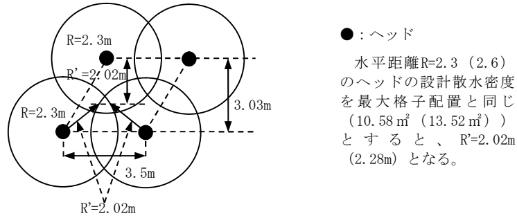
第3-12図 散水密度が低下しないようにした千鳥型配置の例
